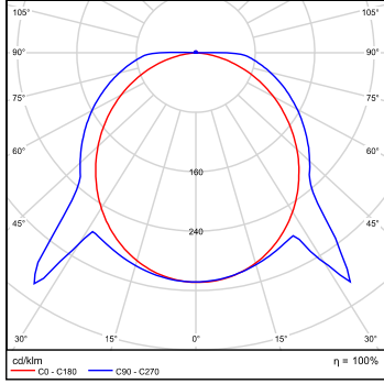
Işık Yayımlı 1 - Polar LVK Light Light Emission 1 - Polar LVK
