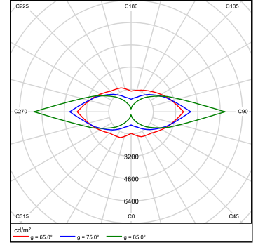
Işık Yayımlı 1 - Işıklık Diagramı Light emission 1 - Skylight Diagram
