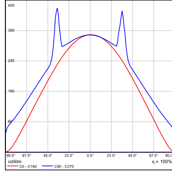
Işık Yayımlı 1 - Lineer LVK Light emission 1 - Polar LVK
